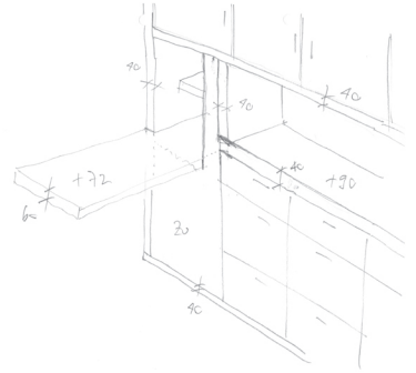
DETAILSKIZZE
